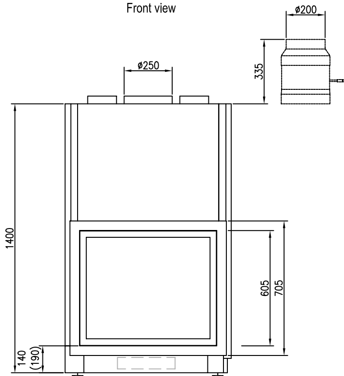
Vooranzicht Frontansicht Vue de face Front view
