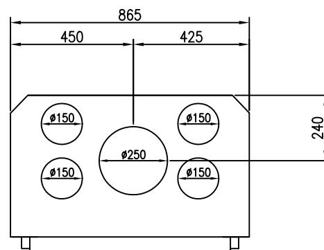
Bovenaanzicht Draufansicht Echangeur Top view
