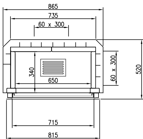
Doorsnede verbrandingskamer Grundriss Feuerstelle Coupe sur foyer Cross section
