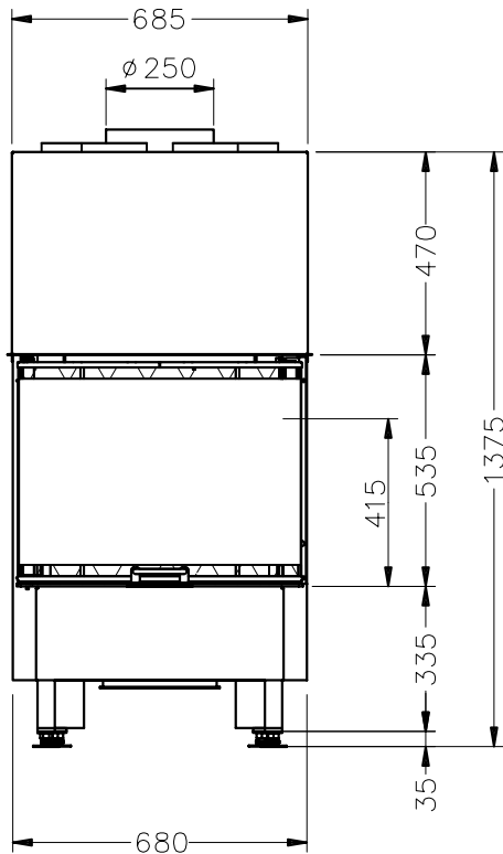
Doorsnede verbrandingskamer Grundriss Feuerstelle Coupe sur foyer Cross section
